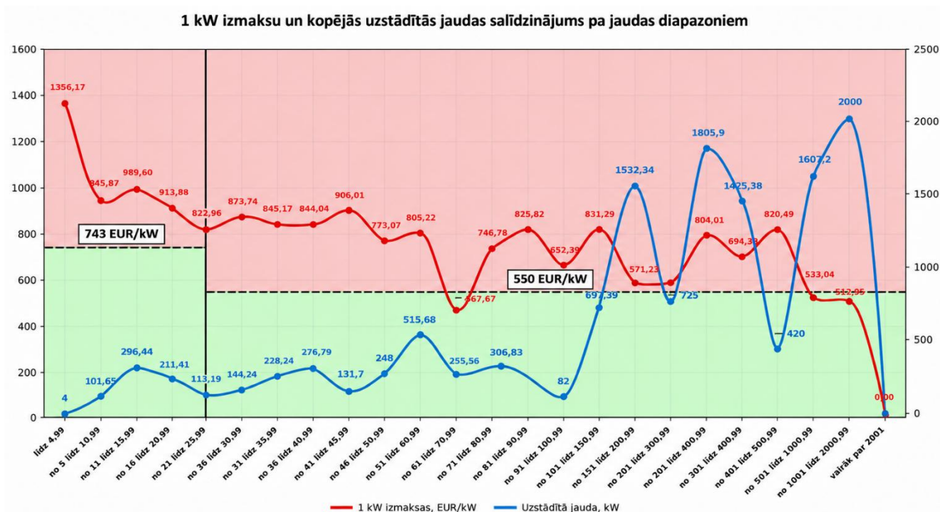
7. att. Saules paneļu sistēmu 1 kW izmaksu un uzstādītās jaudas salīdzinājums pa jaudas diapazoniem atbilstoši noteiktajām likmēm
