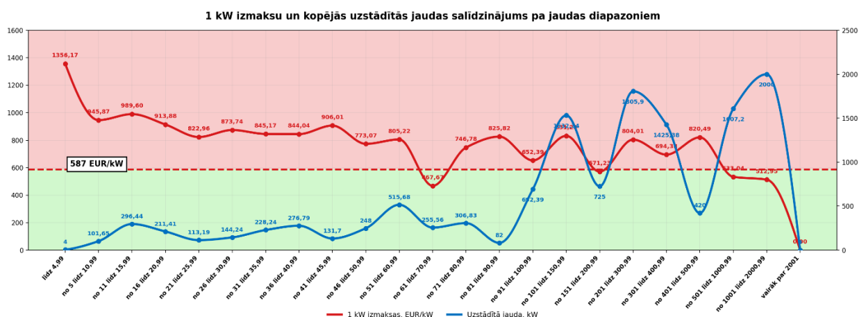
5. att. Saules paneļu sistēmu 1 kW izmaksu un uzstādītās jaudas salīdzinājums pa jaudas diapazoniem, piemērojot 587 EUR/kW robežvērtību
