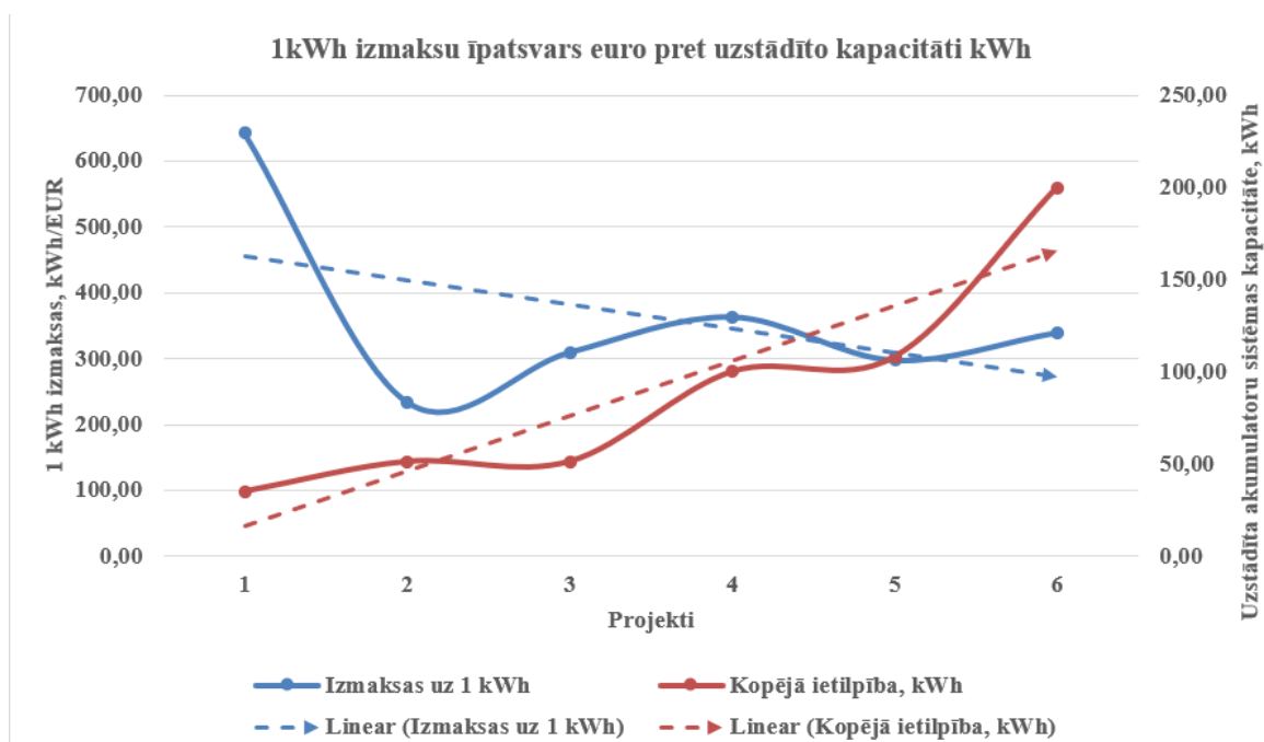
2. att. Elektroenerģijas akumulējošo sistēmu 1 kWh izmaksu un uzstādītās ietilpības savstarpējā sakarība
