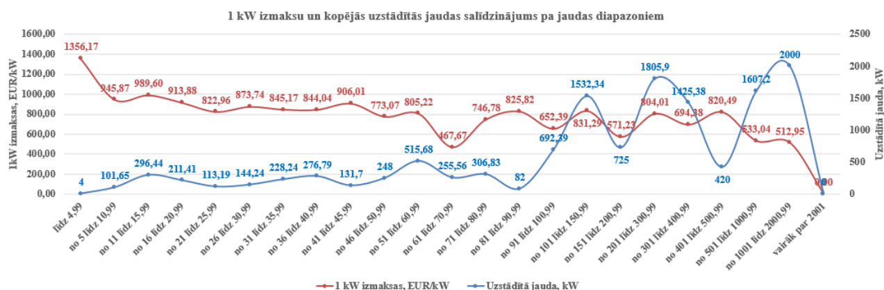
3. att. Saules paneļu sistēmu 1 kW izmaksas un kopējā uzstādītā jauda pa jaudas diapazoniem
