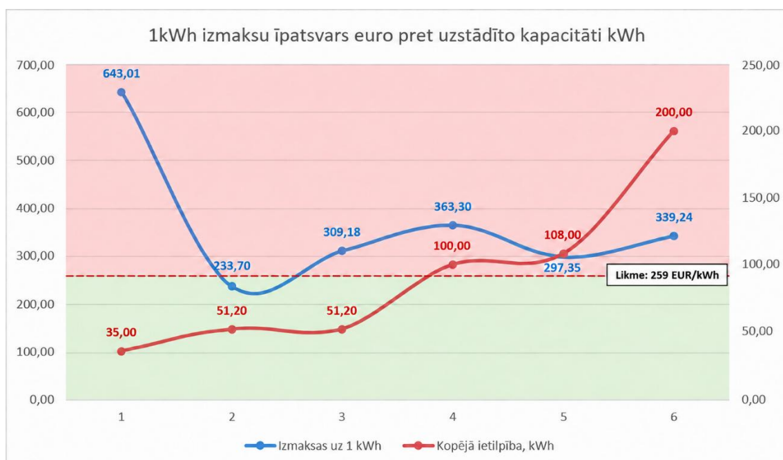
6. att. Elektroenerģijas akumulējošo iekārtu 1 kWh izmaksu un uzstādītās ietilpības salīdzinājums attiecībā pret 259 EUR/kWh likmi
