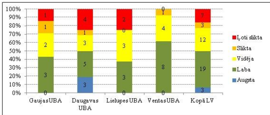
8.attēls. Kopsavilkums par virszemes ūdeņu provizorisko ekoloģisko kvalitāti ūdens objektos Latvija upju baseinu apgabalos 2010.gada vasaras un rudens sezonā. Avots: LVĢMC Ziņojums par virszemes un pazemes ūdeņu aizsardzību 2010.gadā
