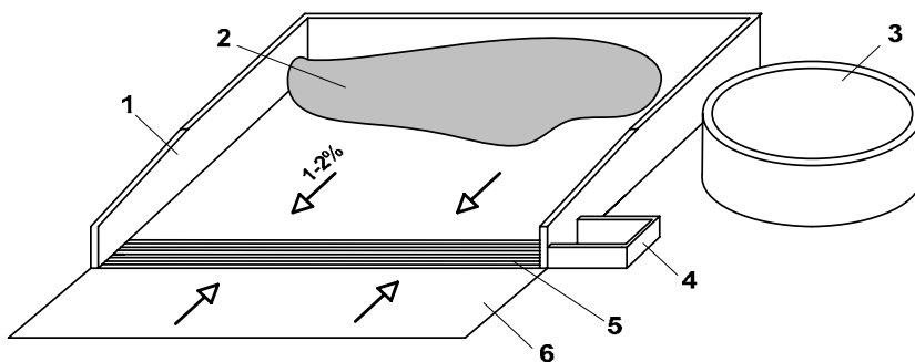
13.2. att. Cieto pakaišu kūtsmēsļu krātuves shēma: 1 – apmale; 2 – kūtsmēsļu kaudze; 3 – vircas krātuve; 4 – vircas starpkrātuve; 5 – vircas savākšanas traps, kas pārsegts ar režģi; 6 – betonējums
